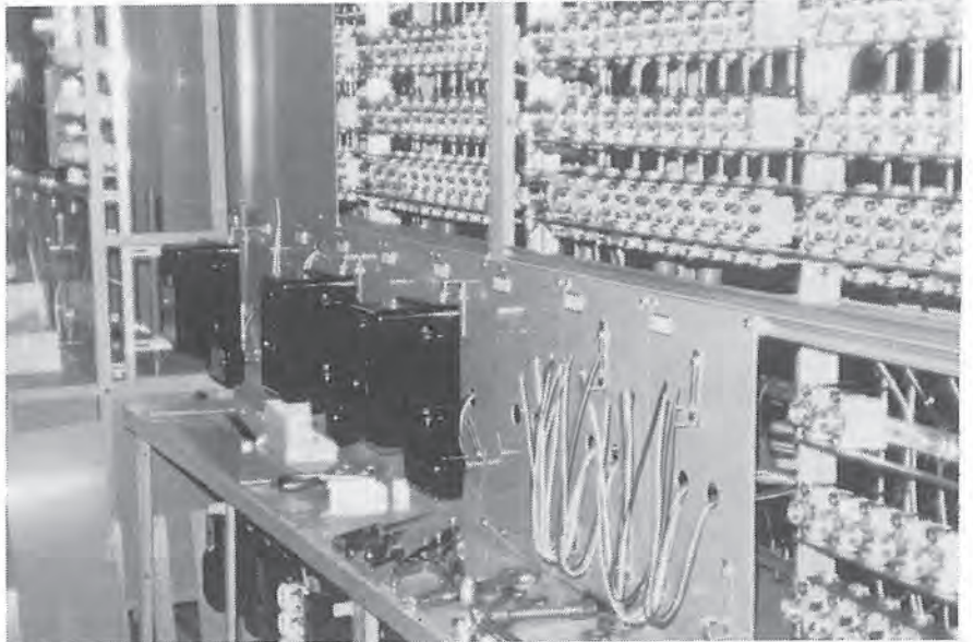
Moderne Hauptverteilung
