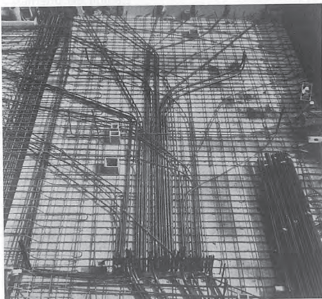
Bis in die 40er Jahre durften in Deckenschalungen nur Panzerrohre verlegt werden. Man stelle sich heute diese Arbeit vor!
