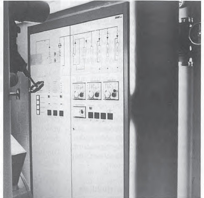
Schalt- und Steuerschrank für die Gesamtanlage mit: - Regelanlagen für Wärmeerzeugung und -verteilung - Kontroll- und Betriebsinstrumenten.
